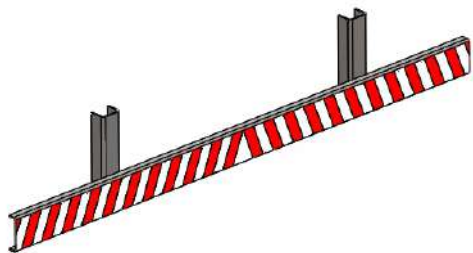
Para-choque HR 21.00.040
