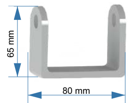
Cavalete Reto 10.02.010
