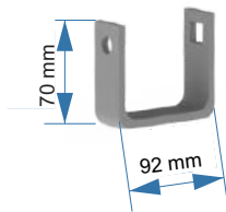
Cavalete Tras. 10.04.011
