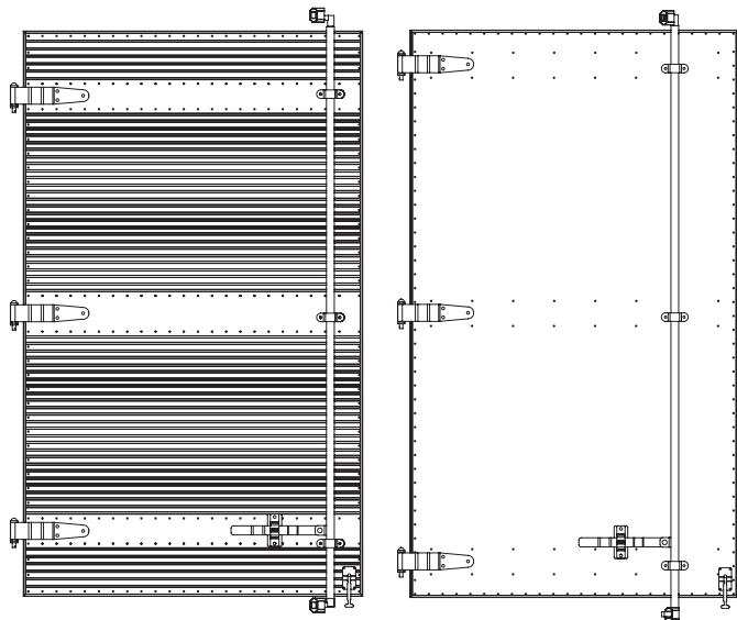
Contorno de Porta 40 mm 99.00.182
