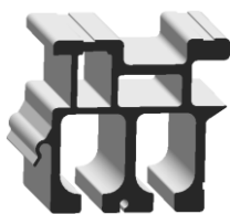
Trilho do Sider RD 99.00.180
