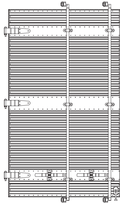
Porta com Varão Duplo
