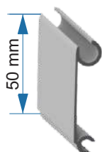
Perfil Intermediario 99.00.417
