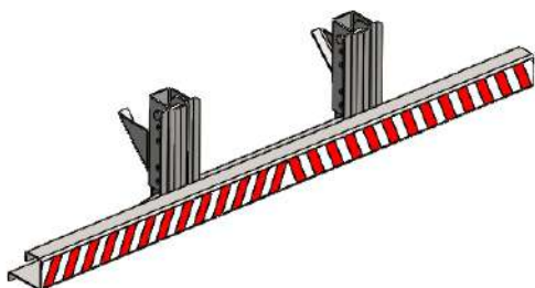
Para-choque 21.00.042
