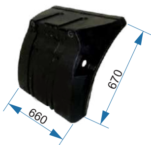
Meio Paralama RD D - 17.07.002 E - 17.07.001
