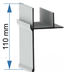
Saia 110 50.04.001
