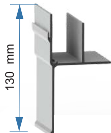
Saia 130 50.01.002
