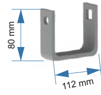
Cavalete largo Tras. Ant. 99.00.172
